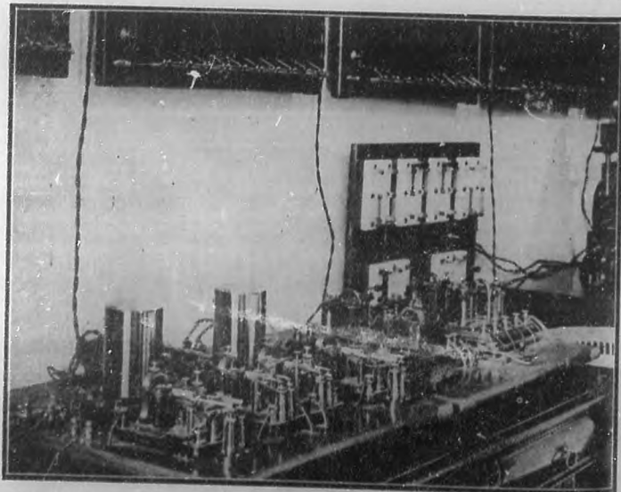
Uno de los aparatos transmisores Musso, para la Telegrafía Rápida por Cables Transoceánicos.
